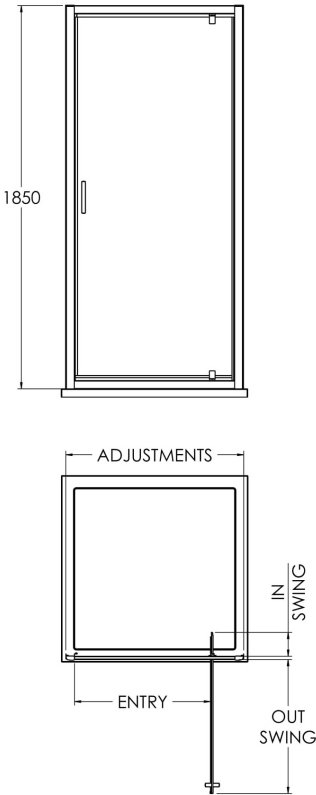
SQ Pivot Door Enclosure
